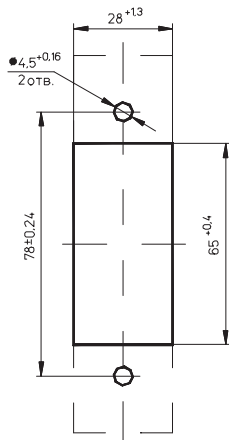
крепление за панель
