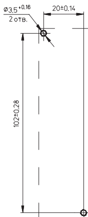
крепление на панель
