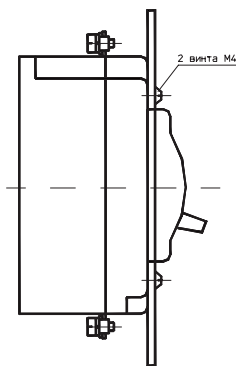
крепление за панель
