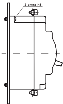
крепление на панель
