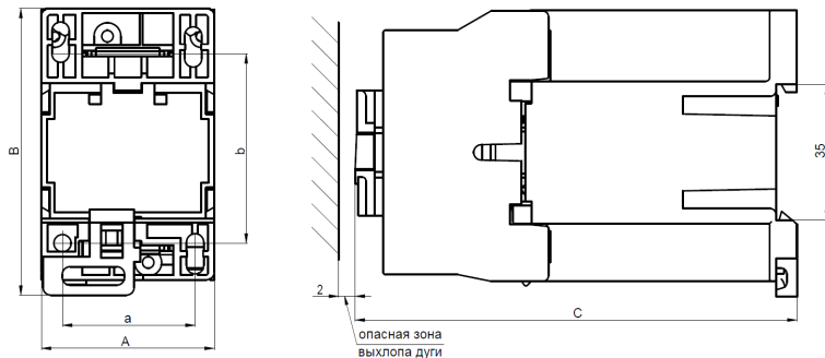
Рисунок А.1. - Контактры нереверсивные на номинальные токи 10, 16, 25, 32 А с управлением на постоянном токе
