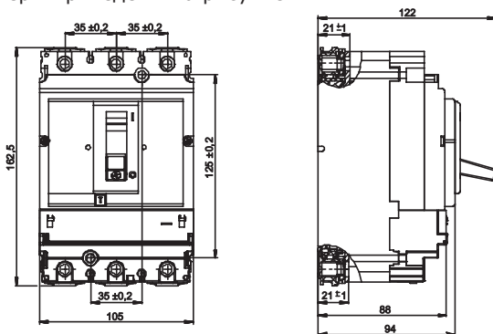
Рисунок 1 - Габаритные, установочные и присоединительные размеры выключателей
